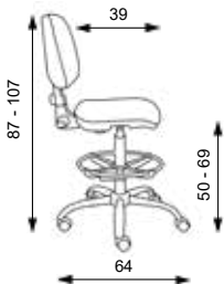
(výška sedadla pri použití vysokého piestu)
