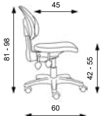
(výška sedu pri použití stoličkového piestu)
