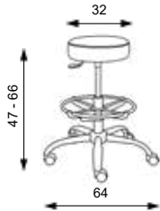
(výška sedadla pri použití vysokého piestu)
