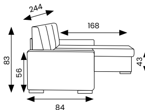
ROZKLADACIA POHOVKA S ĽAVÝM ROHOM / Z POHLADU SEDIACEHO/
