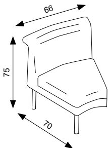
OBLÚKOVÝ DIEL VNÚTORNÝ
